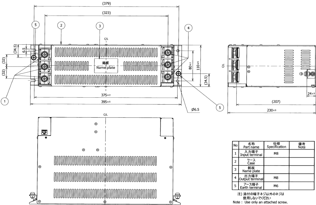
fig. 3 (150A)
