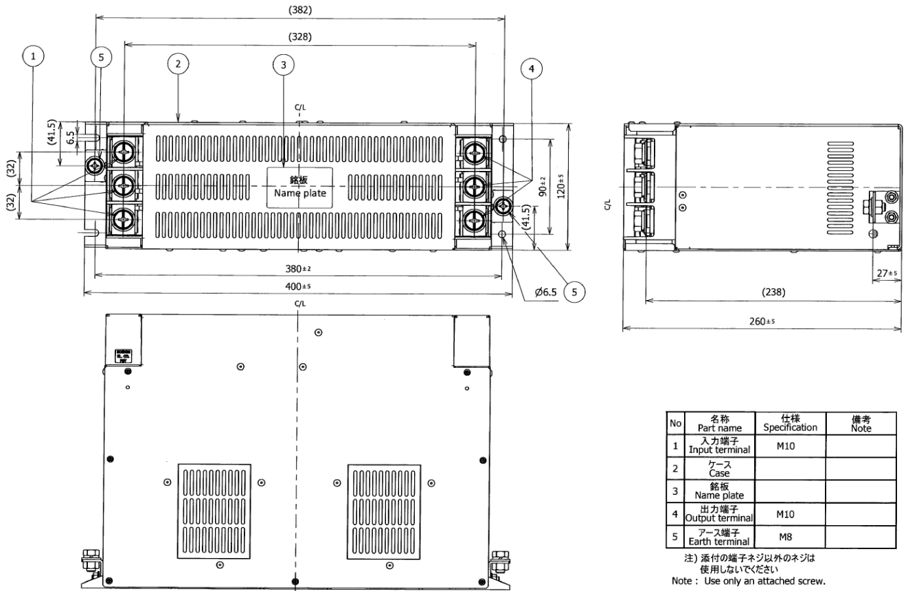
fig. 4 (200~300A)
