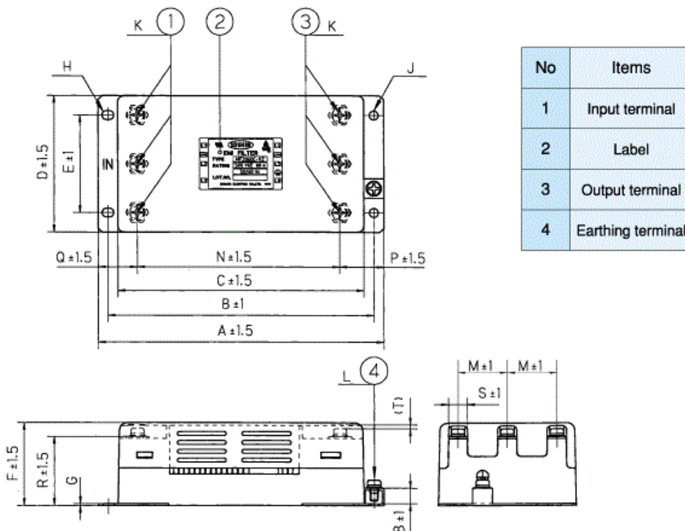
fig.1 (10-60A)
