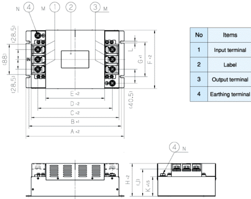
fig.3 (150A)
