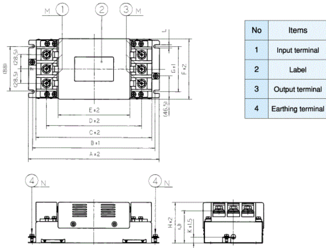
fig.2 (80, 100A)
