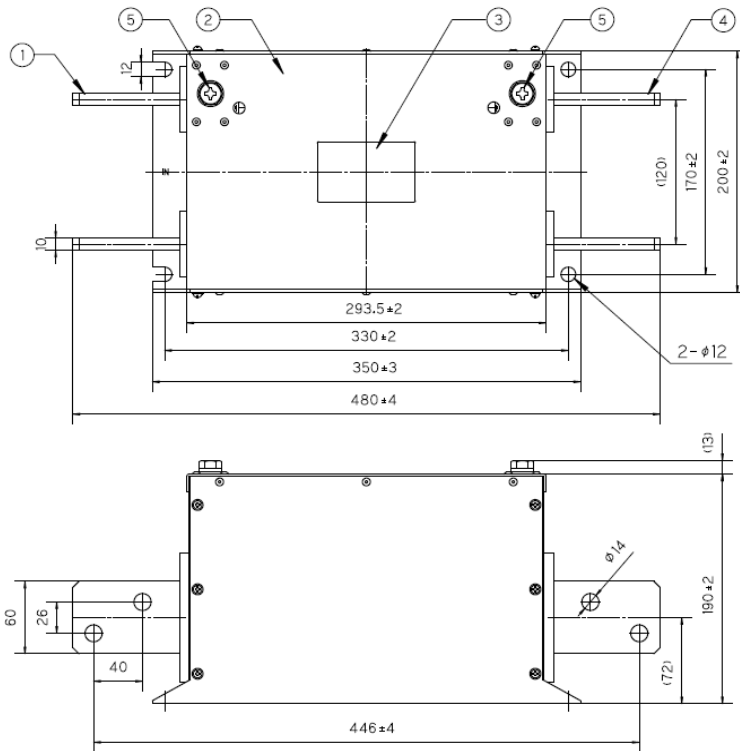
fig.3 (1200A)
