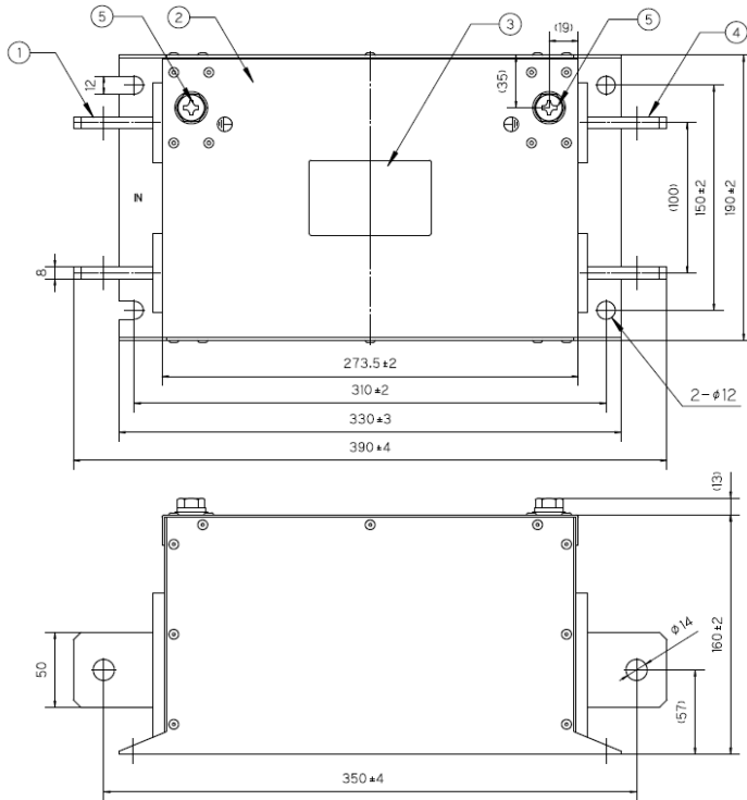
fig.2 (1000A)
