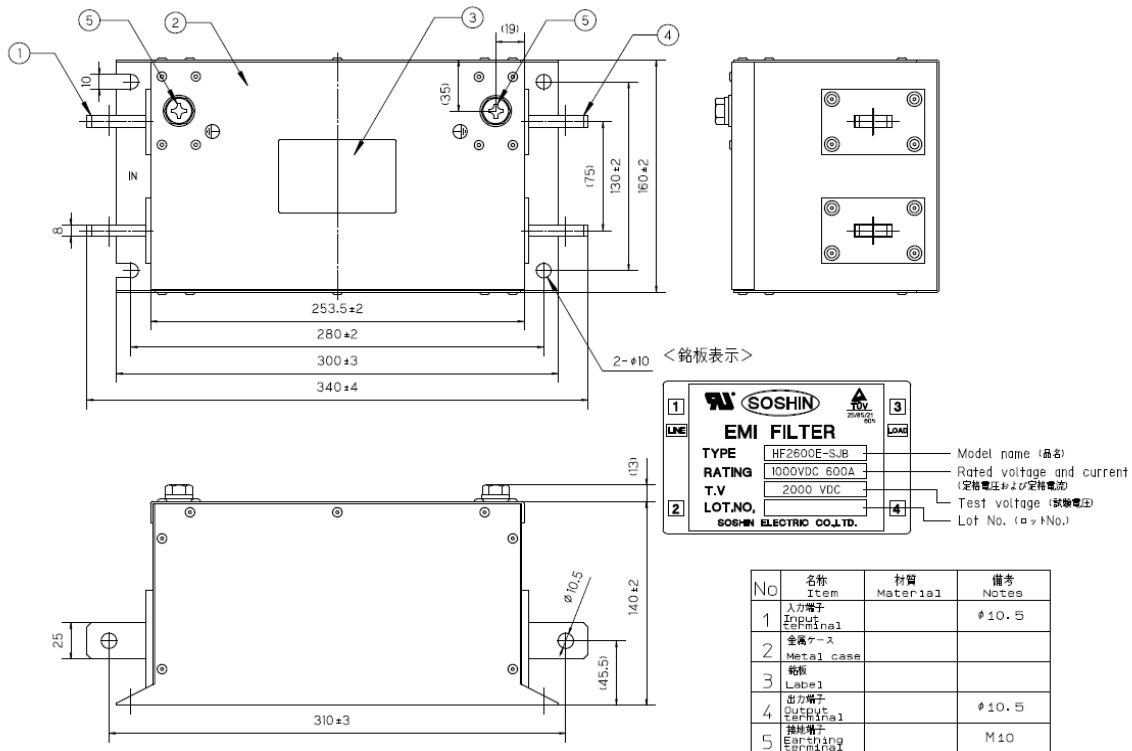
fig.1 (300, 600A)
