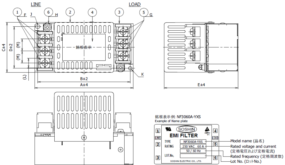
fig.1 (10A~60A)
