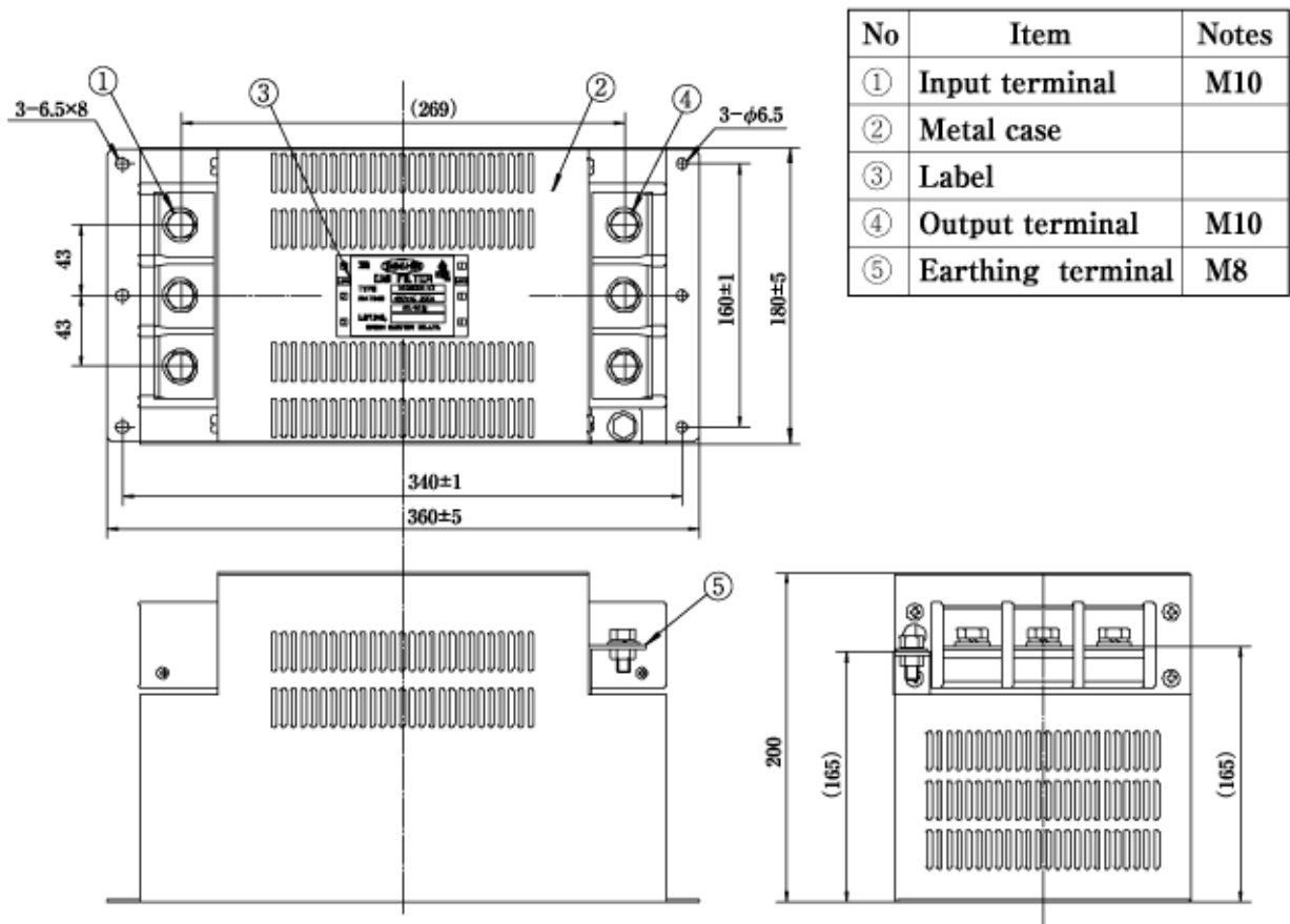
fig. 4 (200, 250, 300A)
