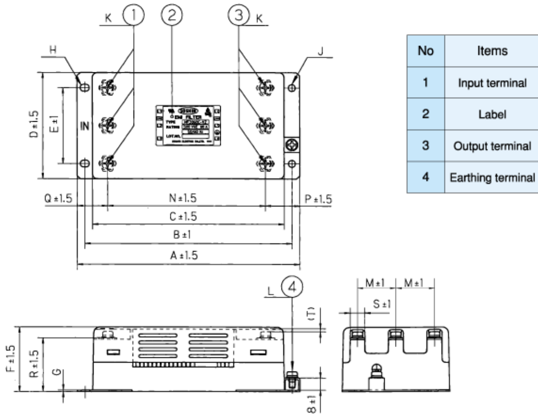
fig. 2 (80, 100A)
