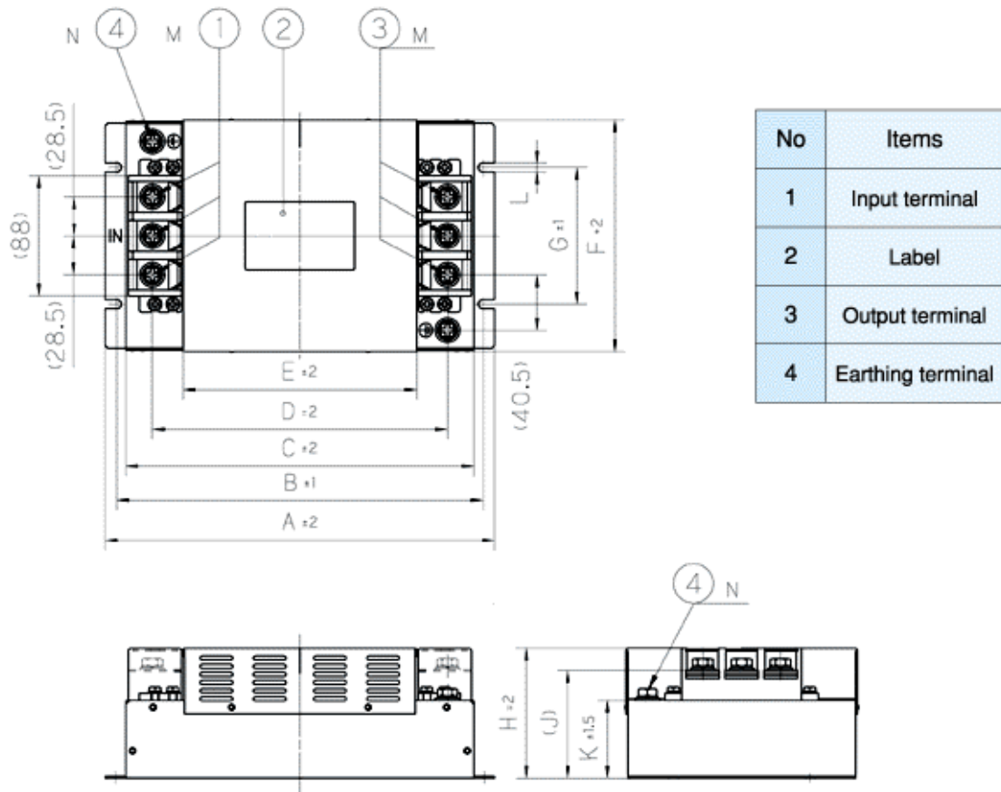
fig. 3 (150A)
