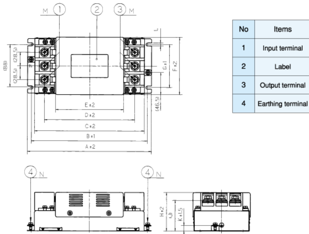
fig. 2 (80, 100A)
