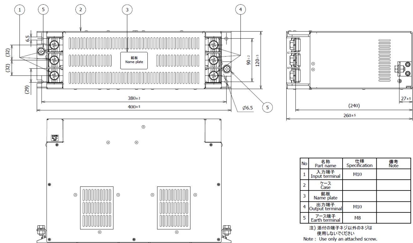
fig. 4 (200~300A)
