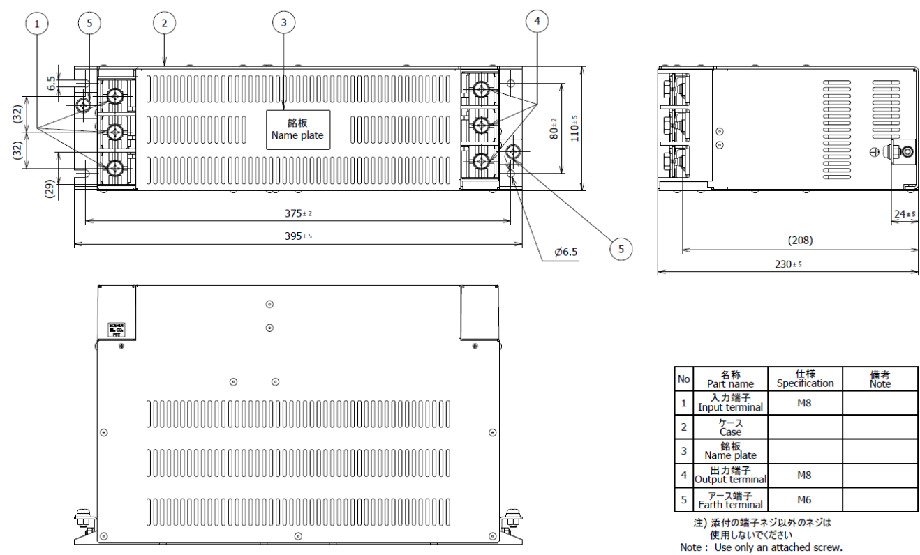
fig. 3 (150A)
