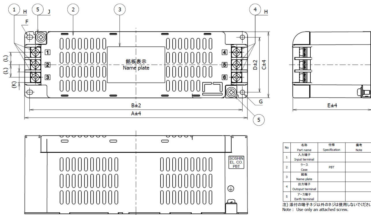
fig.1 (10~60A)
