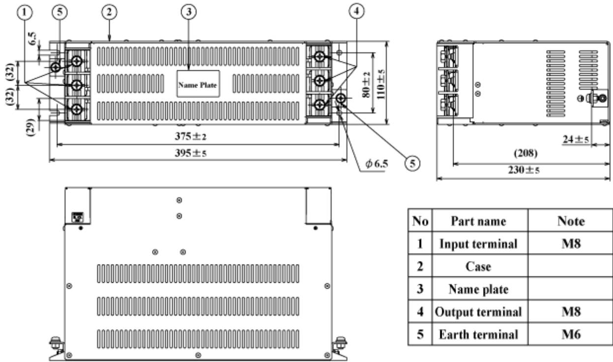
fig.4 (150A)
