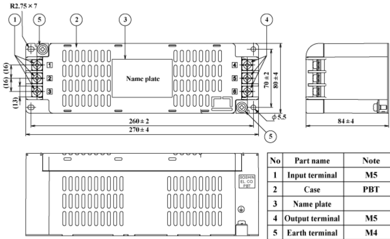
fig.2 (40-60A)
