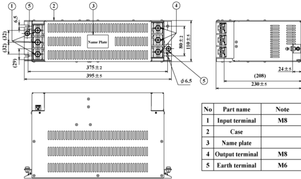
fig.4 (150A)
