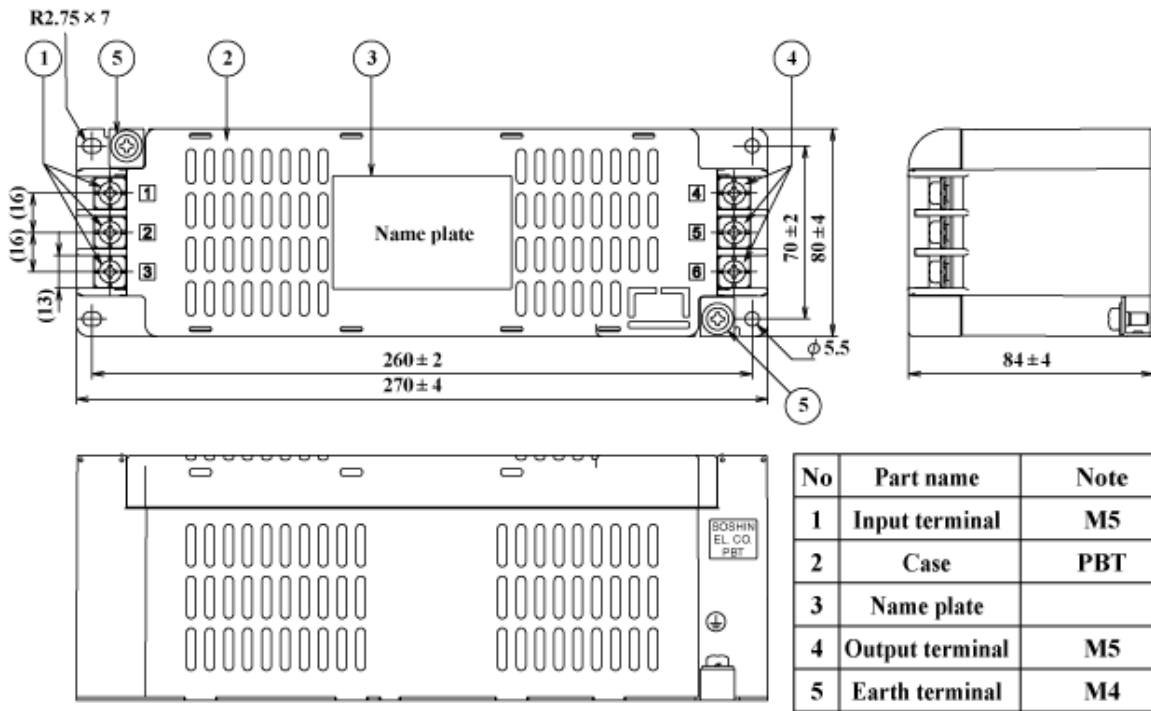
fig.2 (40-60A)
