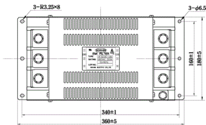
fig. 1 (200, 250, 300A)
