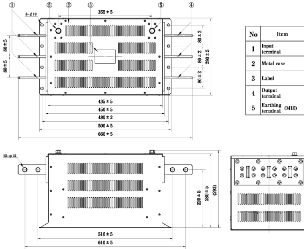
fig. 5 (900, 1000A)
