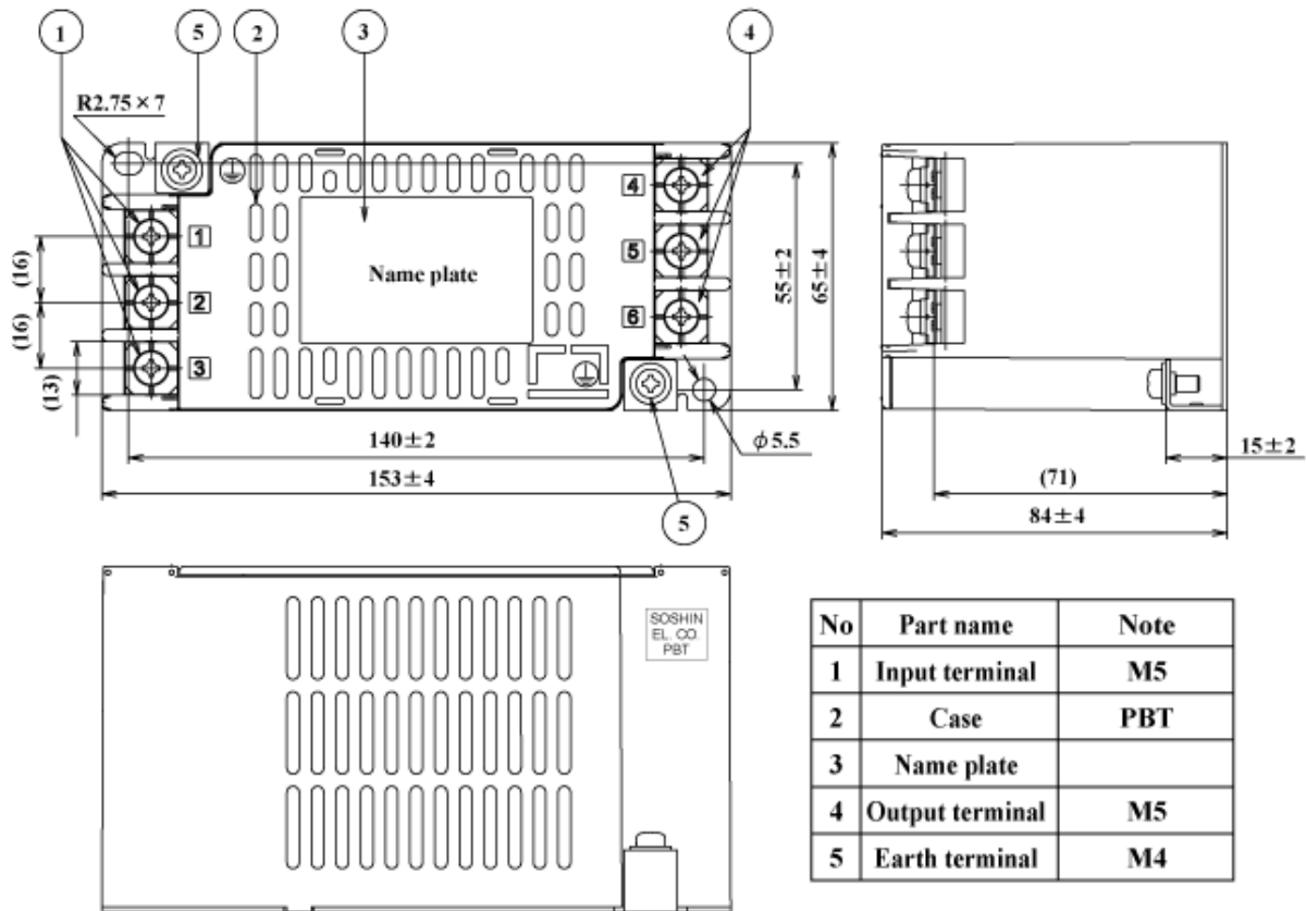
fig.2 (40-60A)
