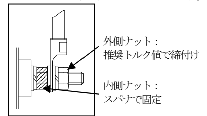
図1. ボルト端子の固定方法
