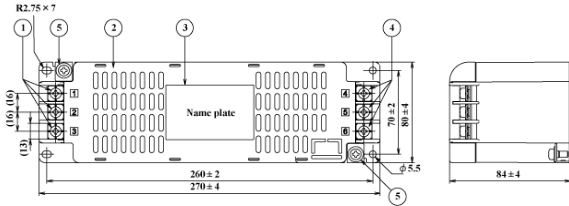
fig.2 (40-60A)
