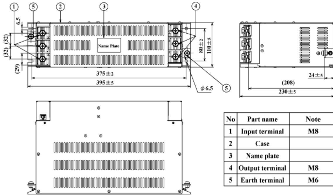
fig.4 (150A)
