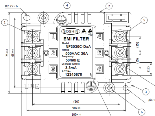
銘板表示例: NF3030C-DxA Example of Name plate
