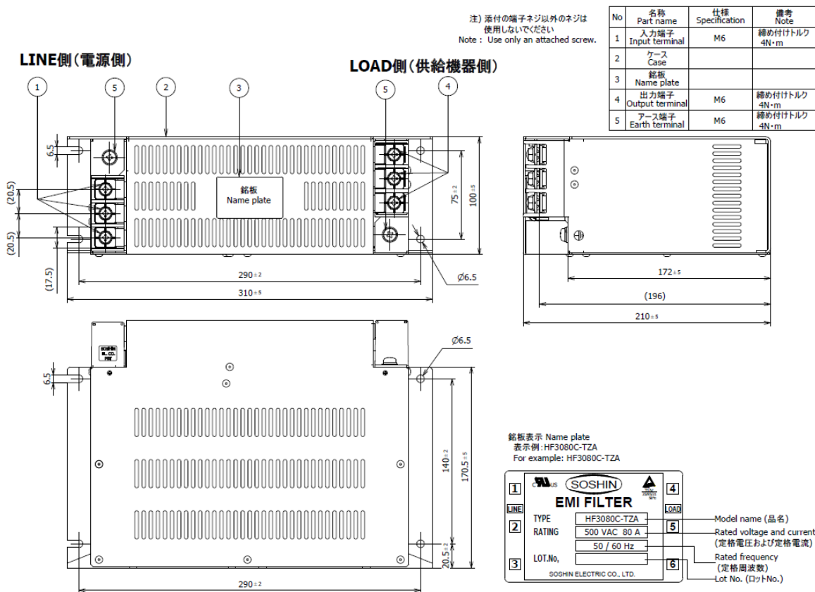
fig.1 (80~100A)
