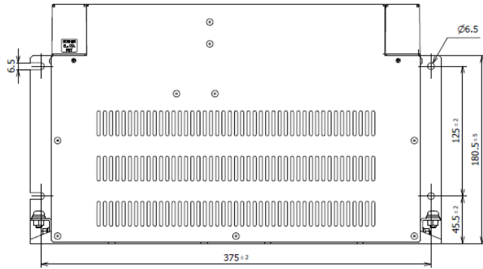
fig.3 (200~300A)
