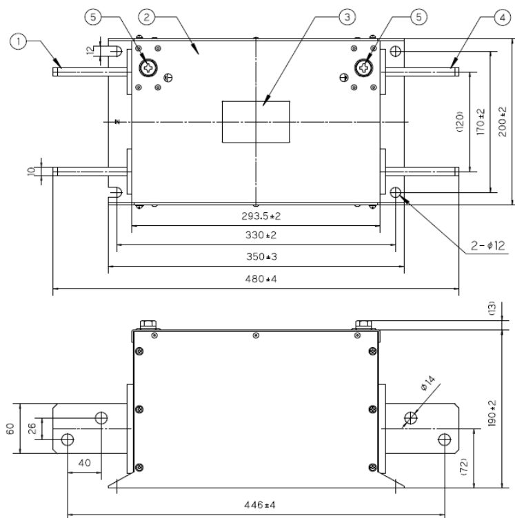
fig.3 (1200A)
