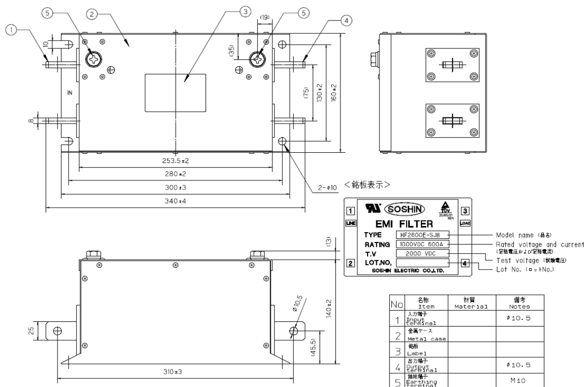
fig.1 (300, 600A)
