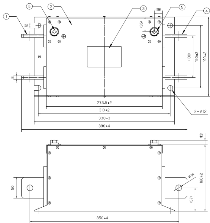
fig.2 (1000A)
