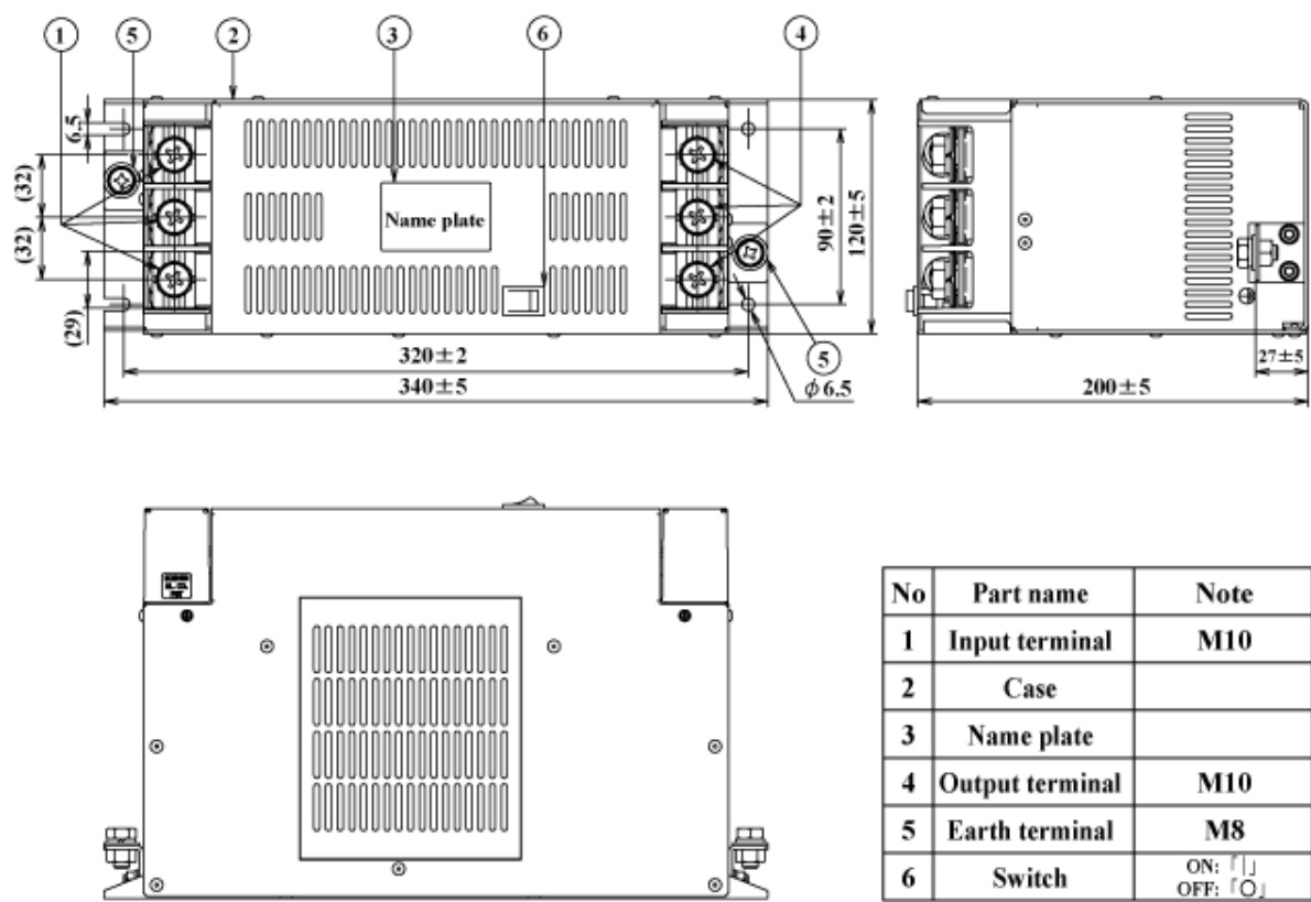
代表特性 (NF3050C-SWA with Switch ON)
