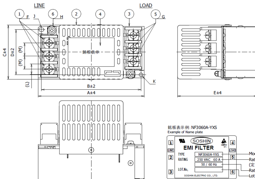
fig.1 (10A~60A)
