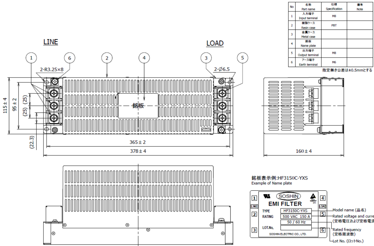
fig.4 (125~150A)
