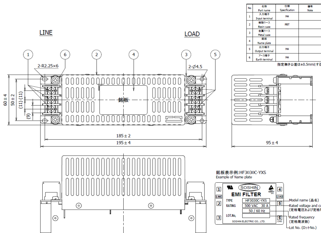
fig.1 (10~30A)
